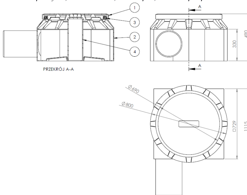
Rys 3. Rysunek zasobnika bez mufy VENKON ZK0 przeznaczony do ułożenia zapasów kabla. 1 – pokrywa, 2 – uszczelka, 3 – korpus, 4 – rura podporowa.
