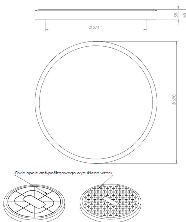
Rys 2. Rysunek i wymiary pokrywy DN690
