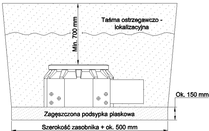
Rys 8. Przykładowe posadowienie zasobnika w gruncie.
