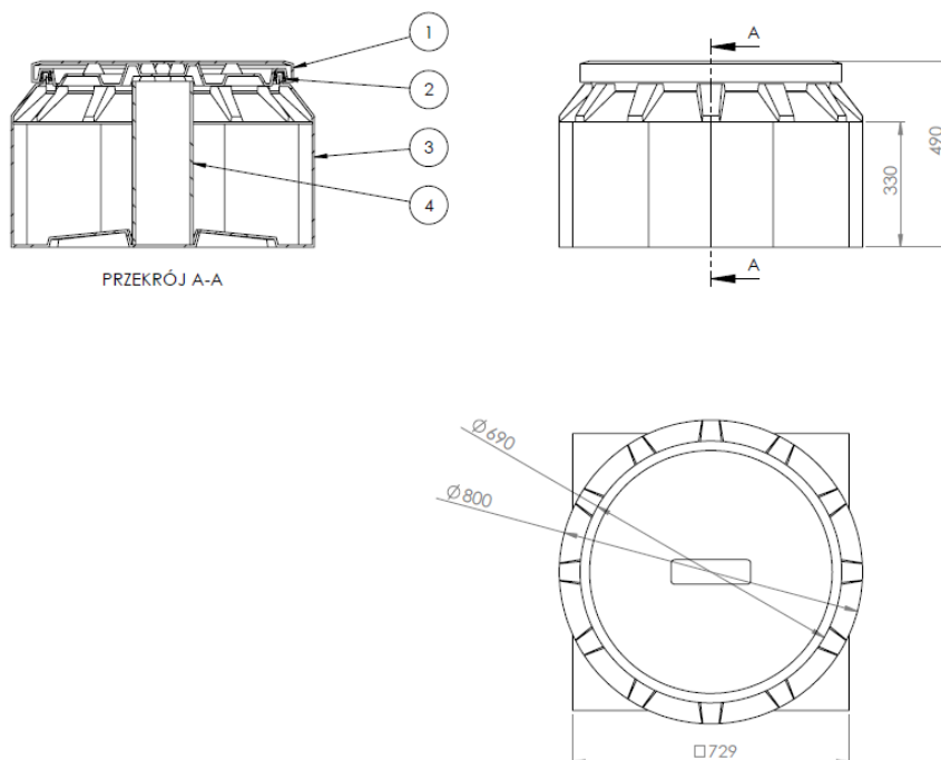
Rys 2. Rysunek i wymiary pokrywy DN690
