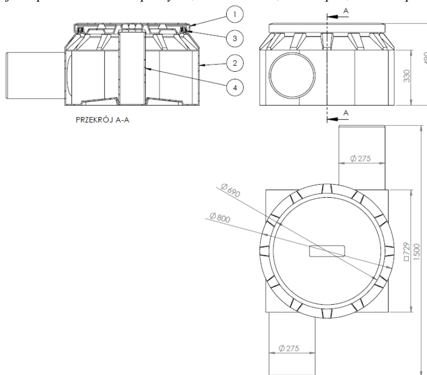
Rys 4. Rysunek zasobnika z jednym miejscem na mufę VENKON ZK1 przeznaczony do ochrony jednej mufy złączowej i zapasów kabla. 1 – pokrywa, 2 – uszczelka, 3 – korpus, 4 – rura podporowa.
