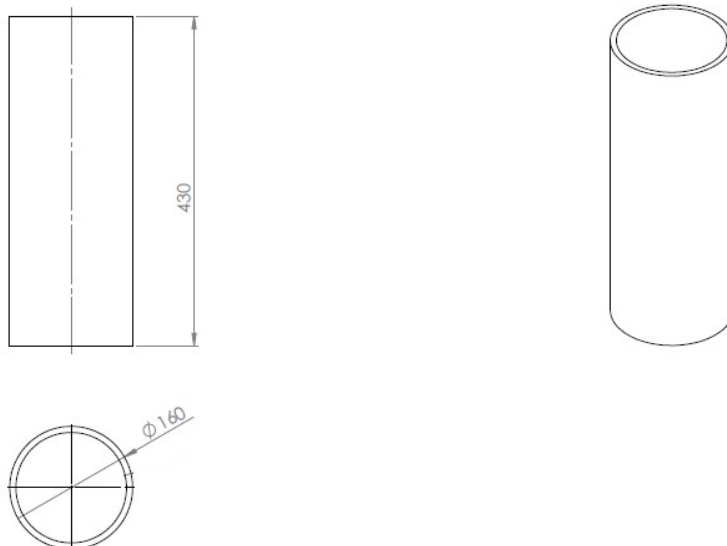
Rys 1. Rysunek i wymiary rury wzmacniającej
