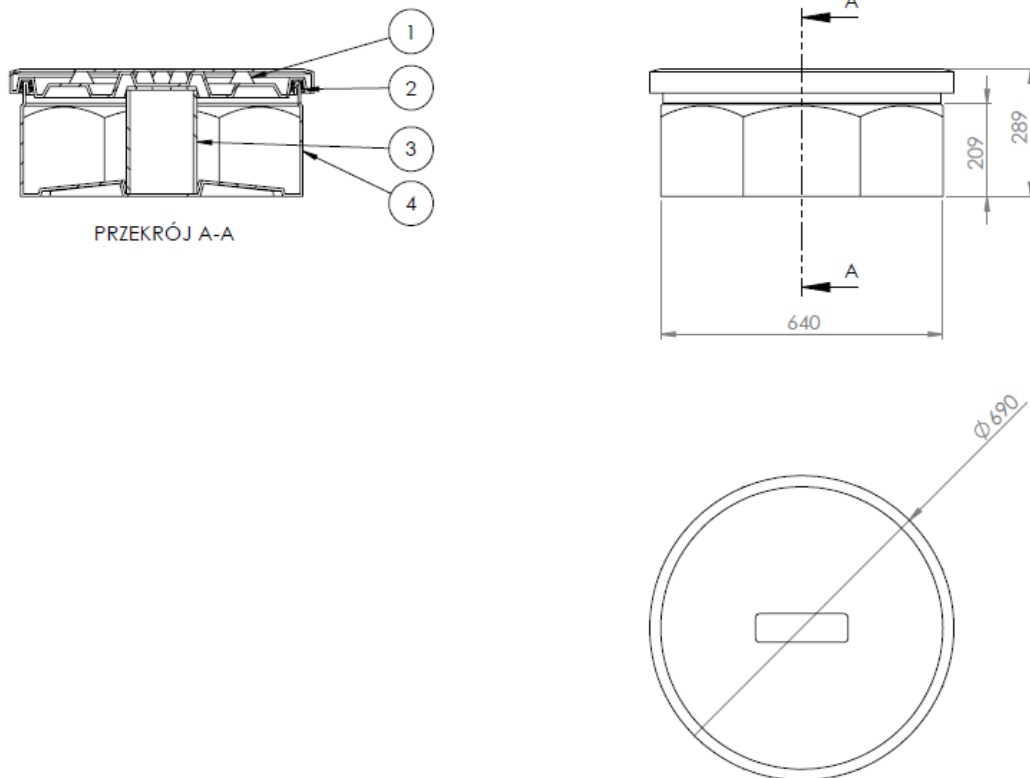
Rys 6. Rysunek zasobnika niskiego VENKON ZKM przeznaczony do ułożenia zapasów kabla. 1 – pokrywa, 2 – uszczelka, 3 – rura podporowa, 4 – korpus.
